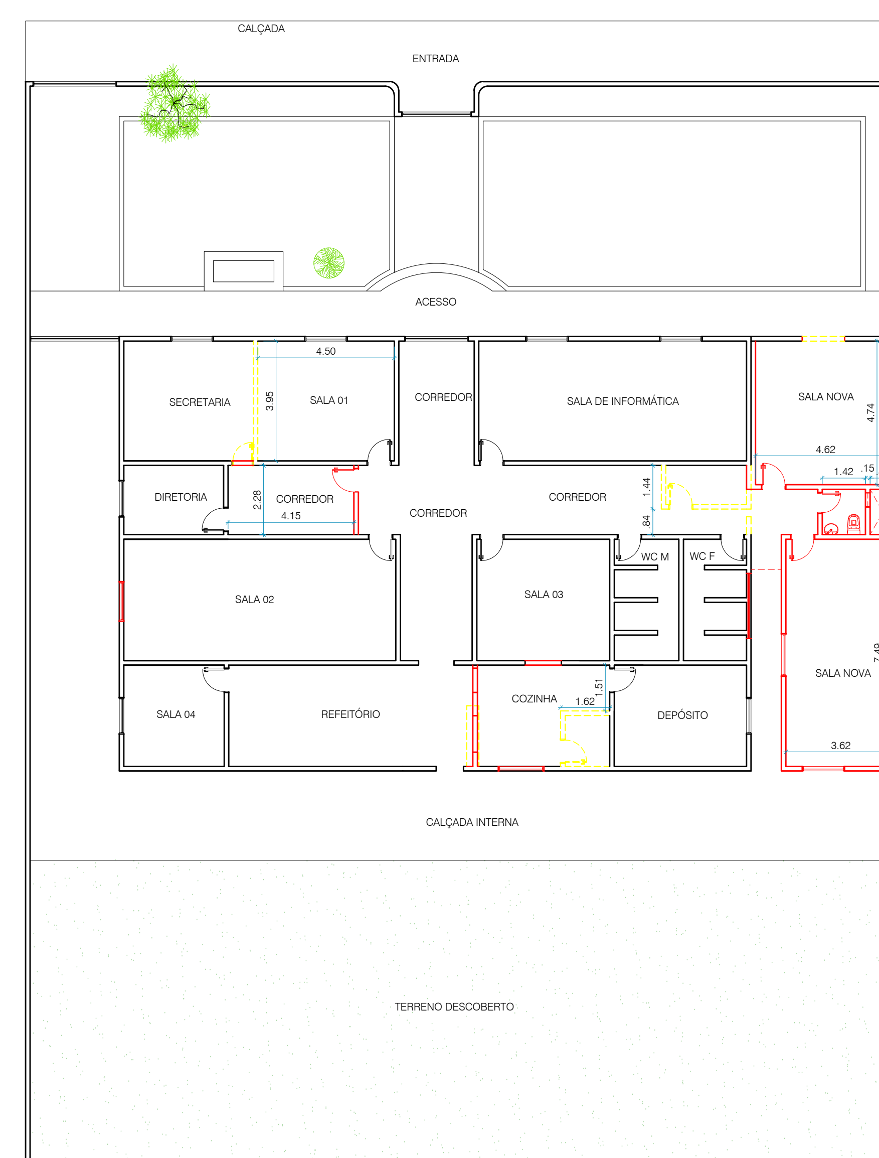
PLANTA BAJXA - REFORMA ESCALA 1:125
